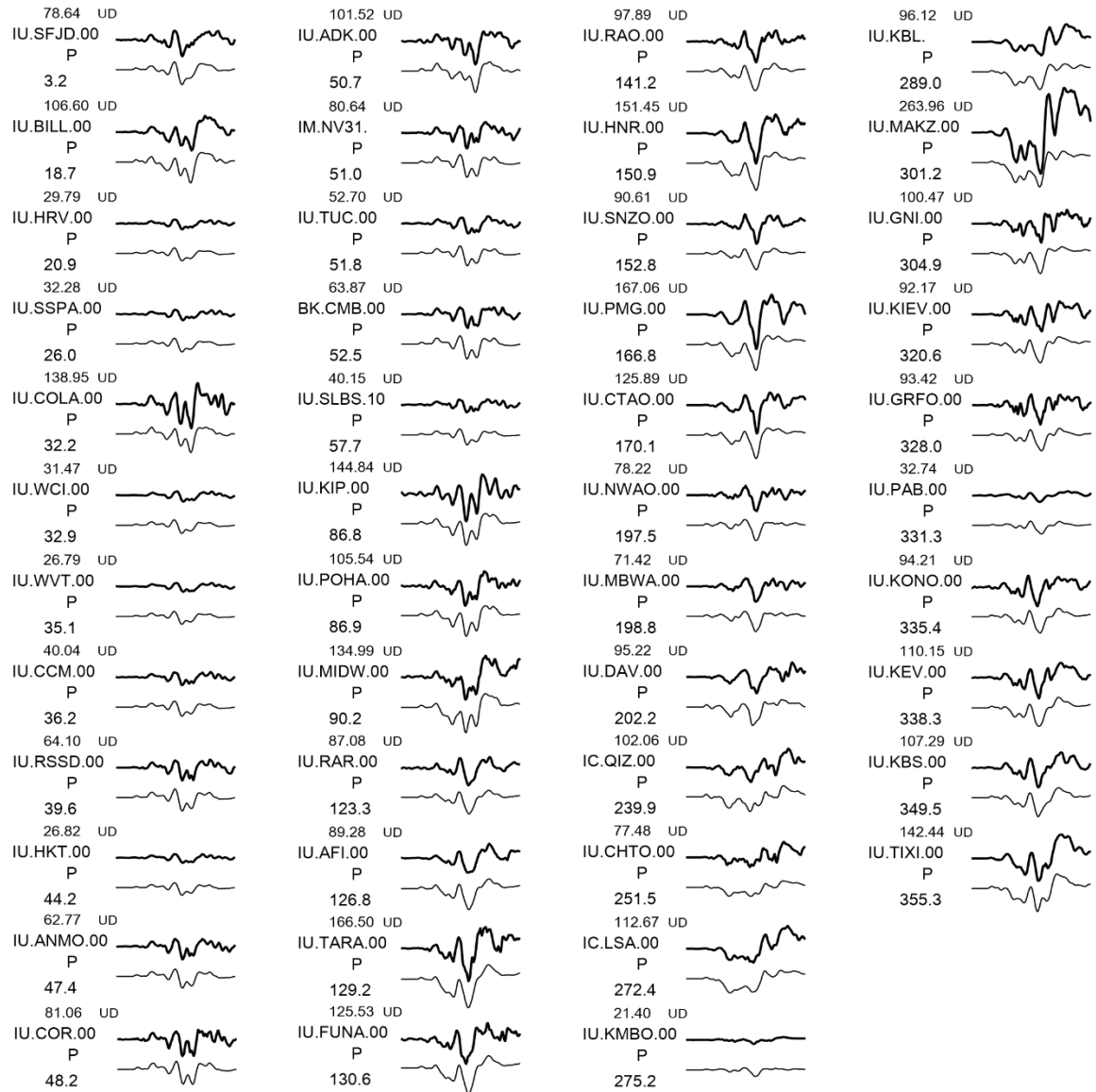
図 1 解析結果 (震源時間関数、メカニズム解、すべり分布、観測波形(上)と理論波形(下))
