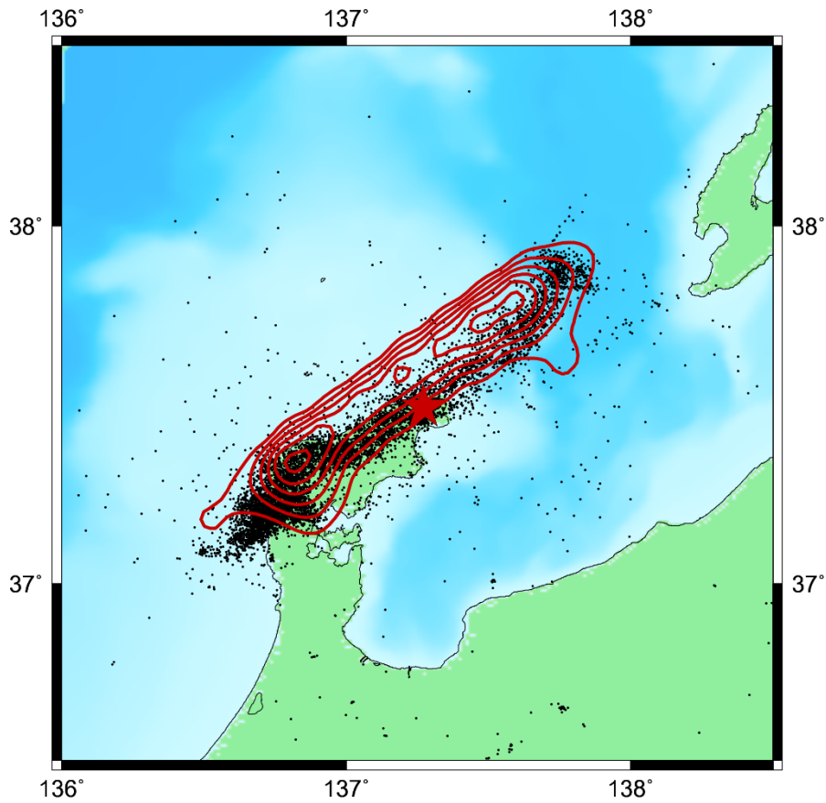
図2 すべり分布(コンター間隔は 0.5m)と1/7 までの余震活動(JMA の速報値による)
