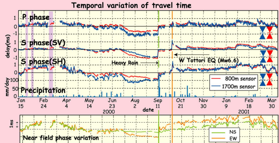
ACROSSの連続観測で捉えた地震波速度の時間変化(淡路島野島断層)
